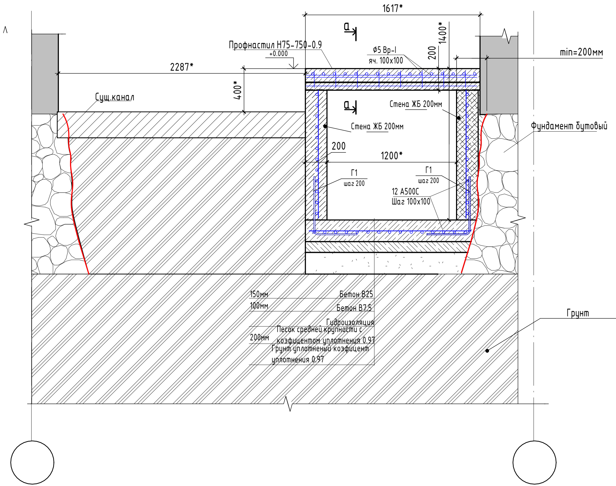
(1-1)(34)Типовой разрез для канала h-низа -1.400 ( 1 : 20)
